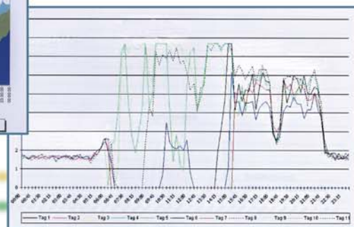
Medición comparativa con ADA entre instalación existente e instalación propuesta
